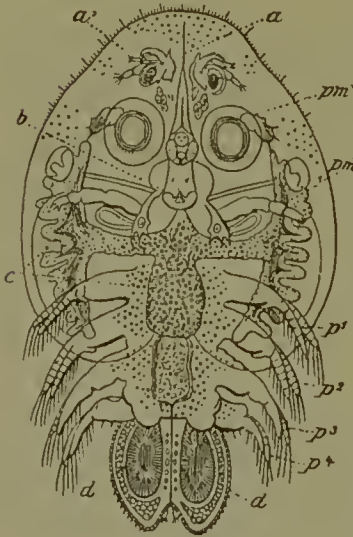
Fig. 96. Argulus foliaceus (natürl Grösse \frac{1}{2} cm).
